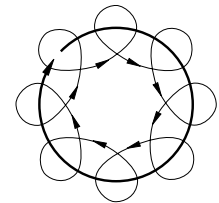
Dia. orbite de 3/16" (5 mm) pour le ponçage général
